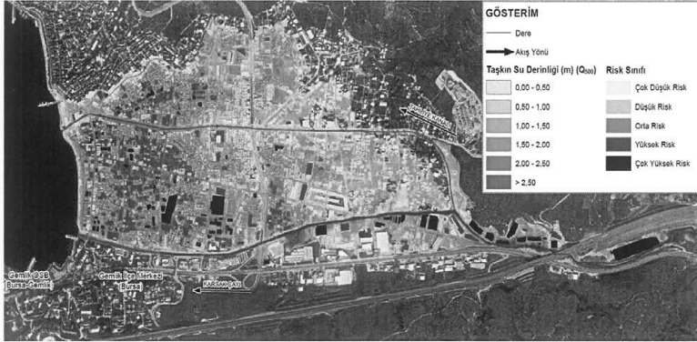
Bursa - Gemlik - Karsak Çayı - Taşkın Risk Haritası
